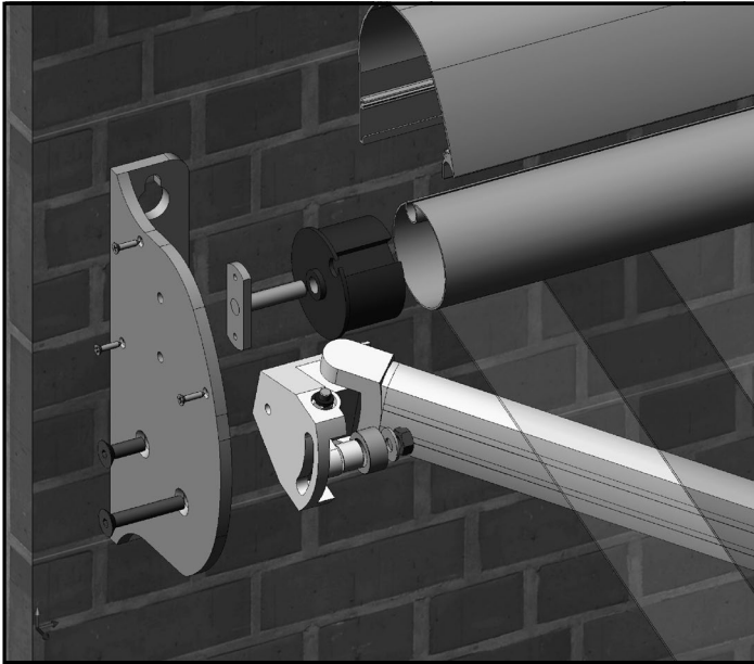
Vivace knikarmscherm 2B
