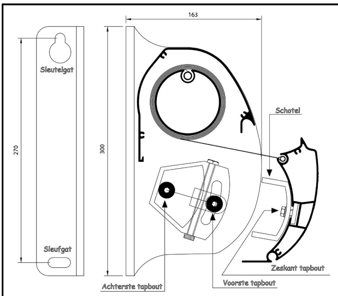
Maatvoering consoles Vivace 2B
