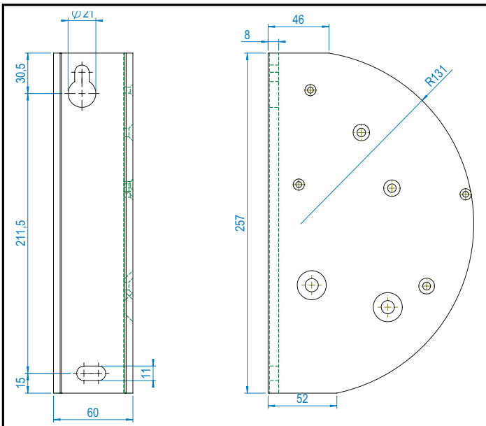
Maatvoering consoles Stanza 2B
