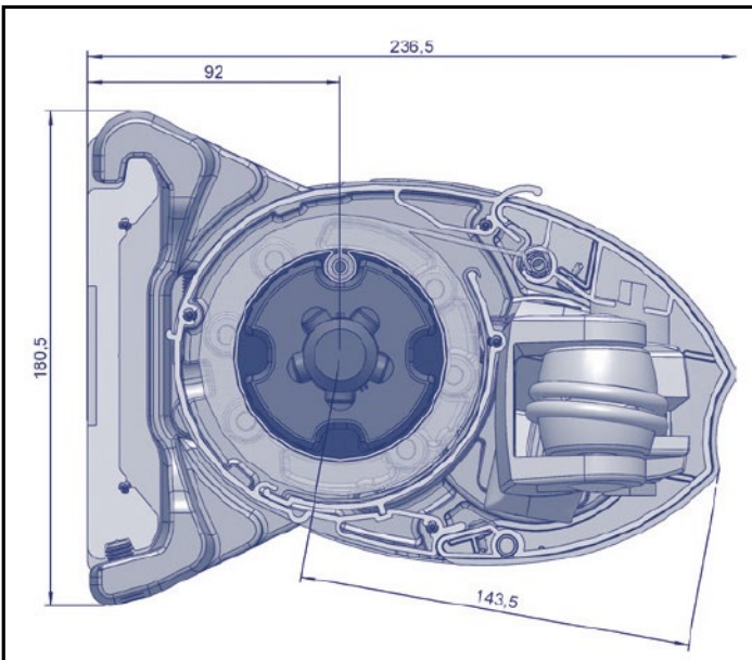
Maatvoering Sopra
