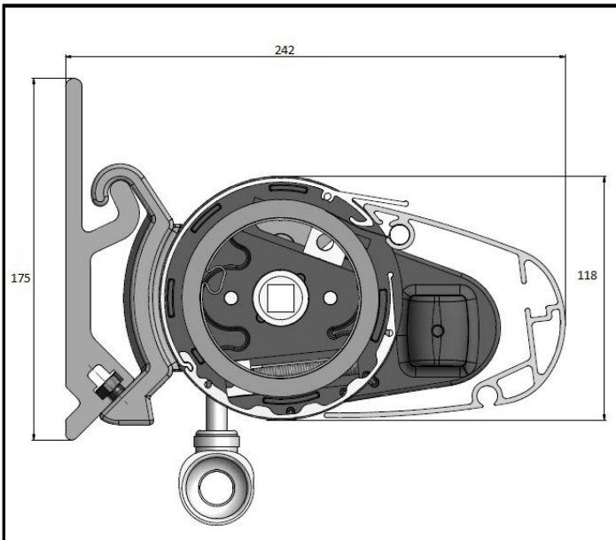
Maatvoering Rondo 2B
