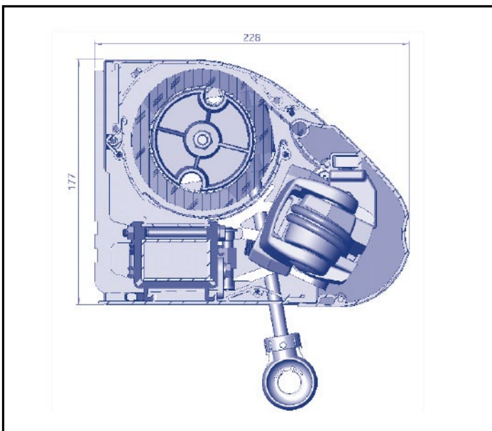
Maatvoering Fuga
