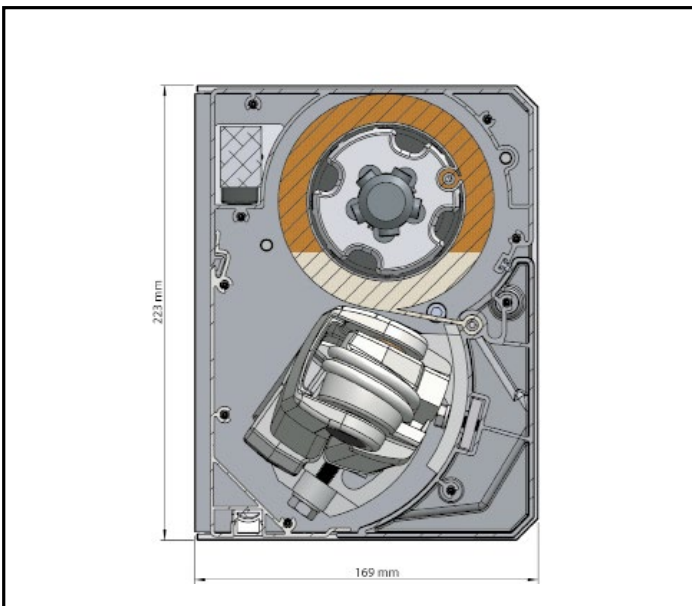
Maatvoering Coda
