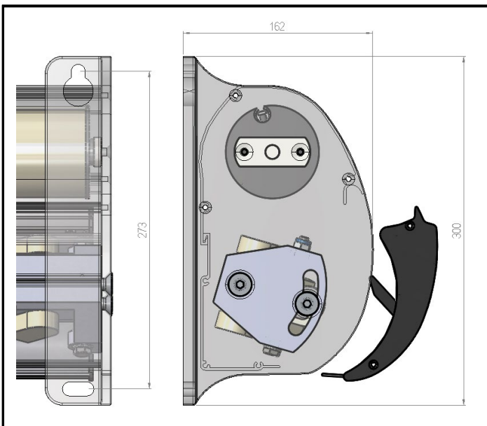
Maatvoering consoles Allegro 2B
